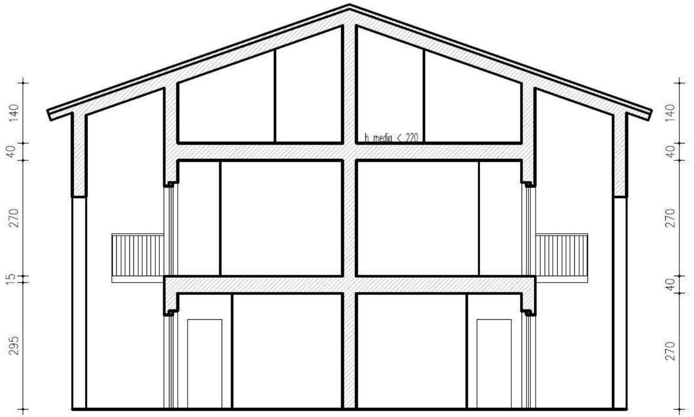
SEZIONE A-A
