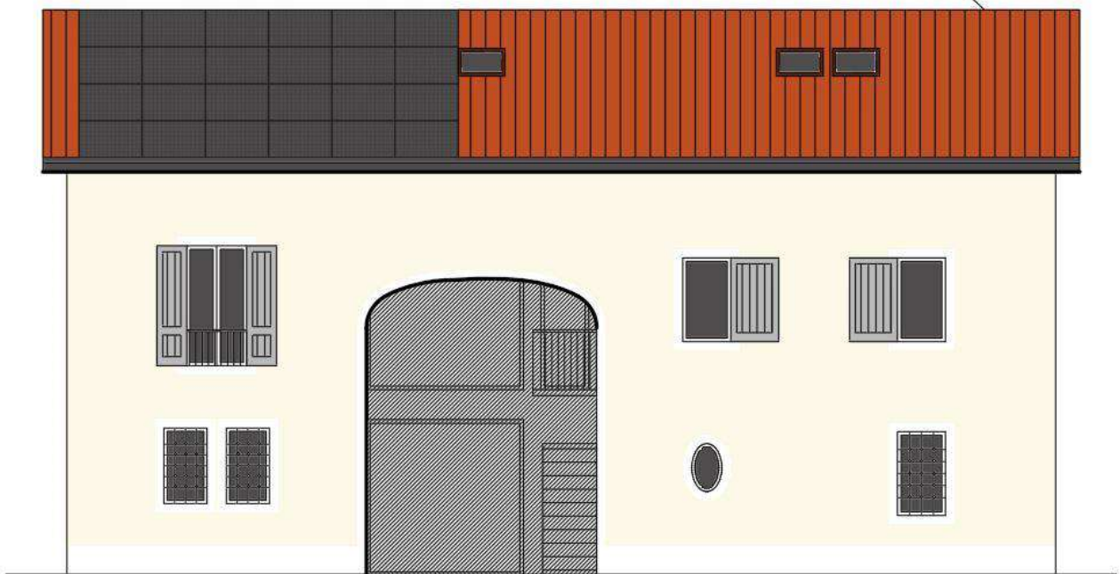
PROSPETTO SUD
