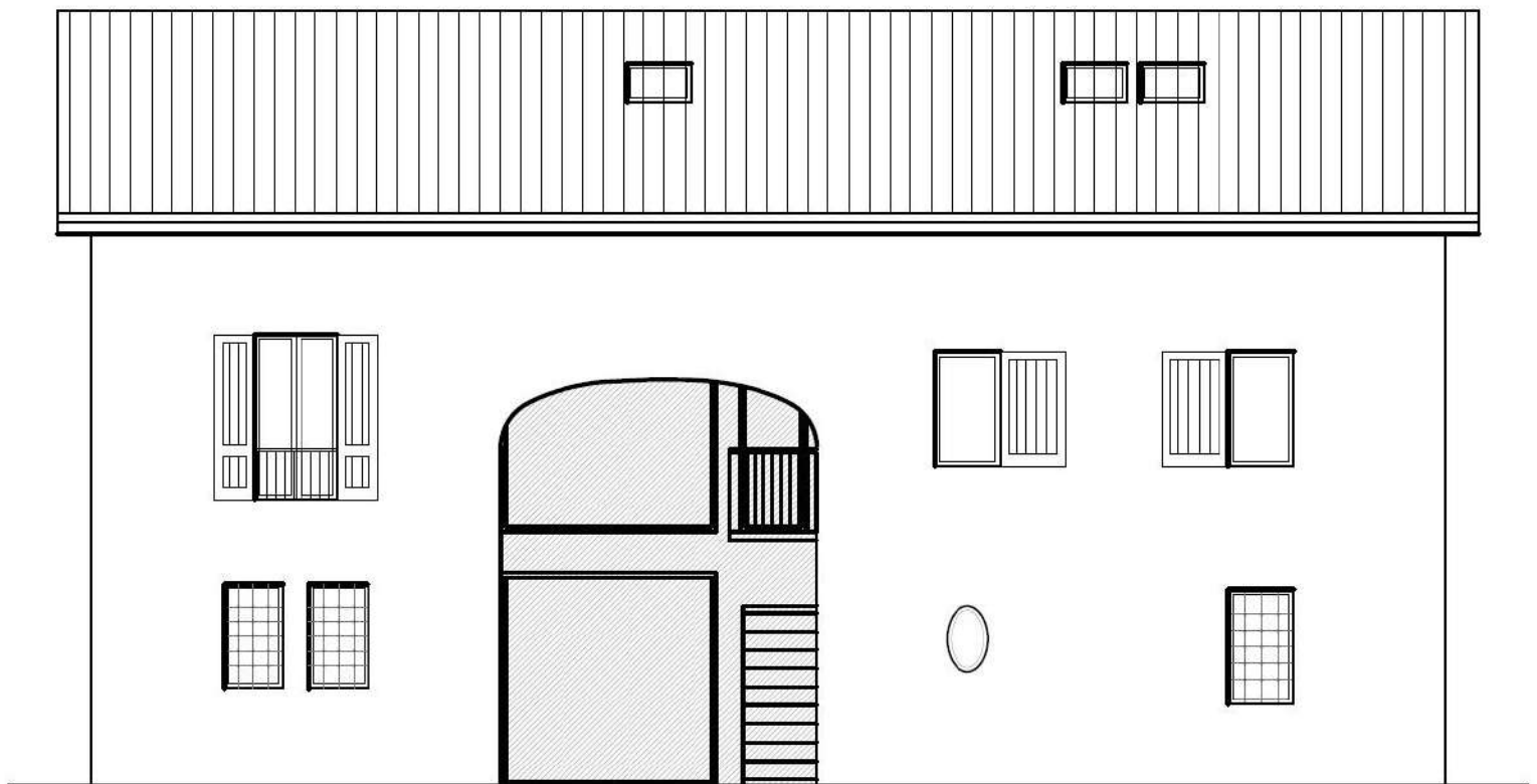
PROSPETTO SUD
