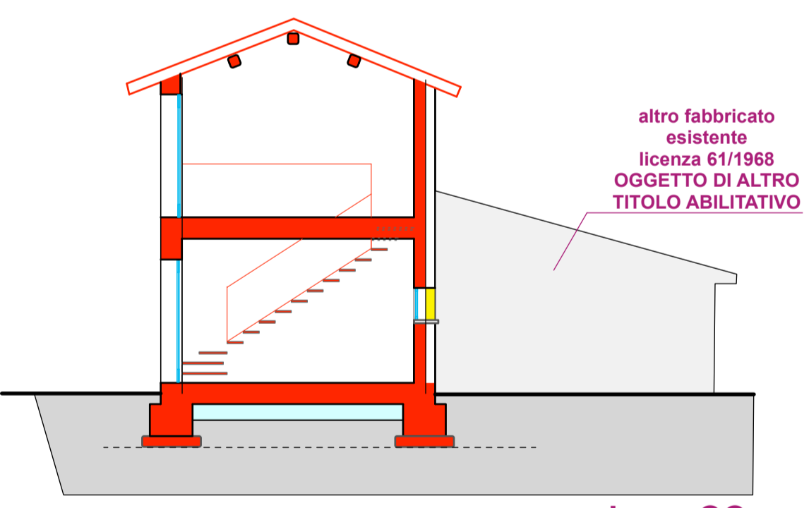
sezione CC
