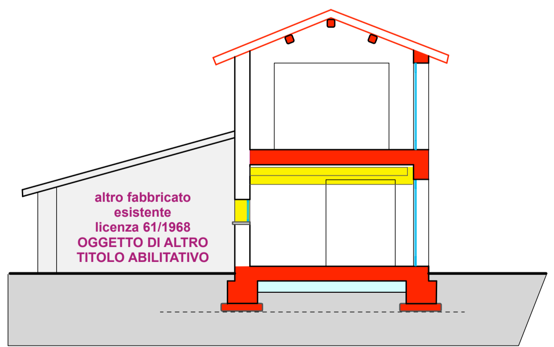
sezione AA
