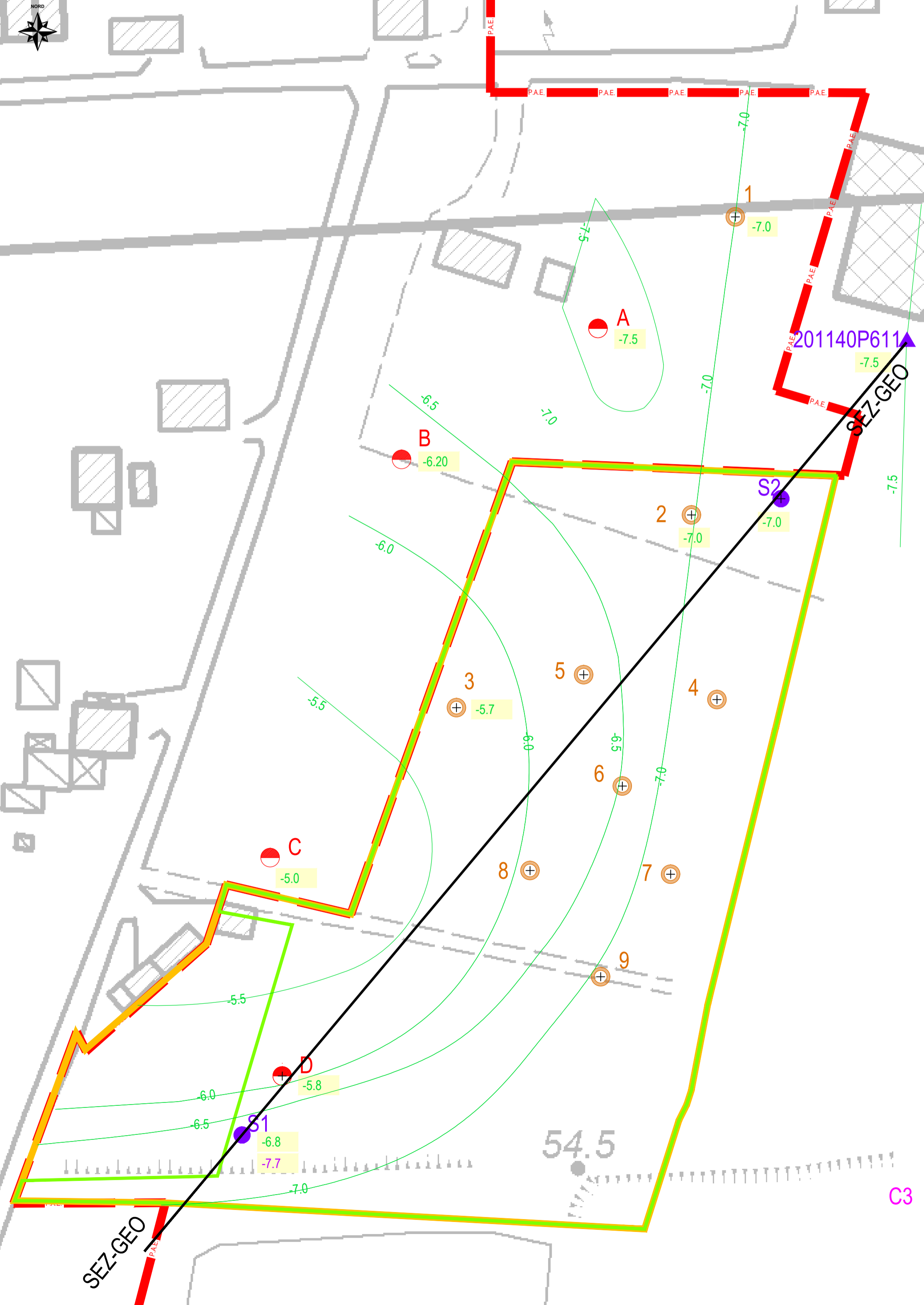
PLANIMETRIA B - SOGGIACENZA DELLA BASE DELLE GHIAIE - scala 1:750
