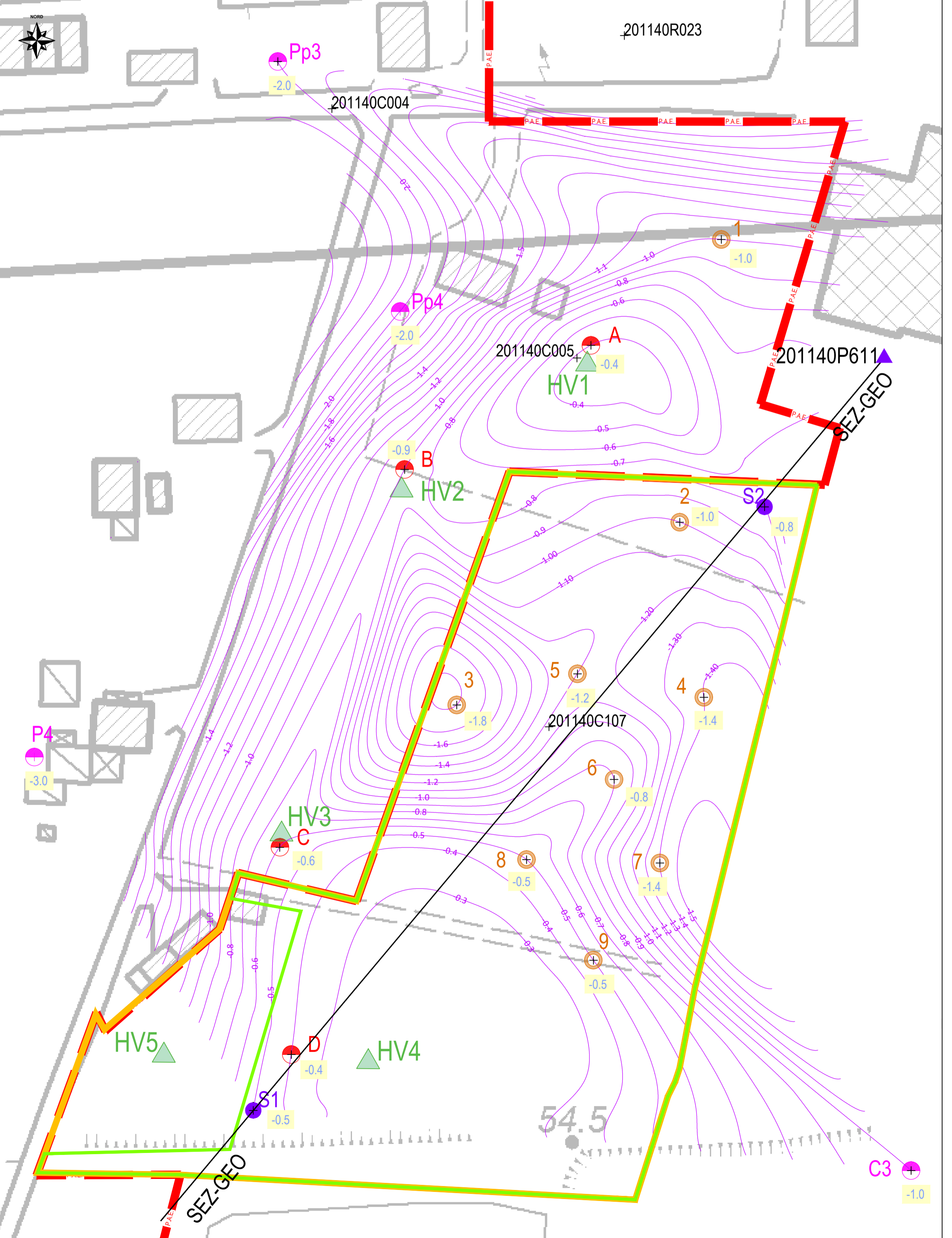
PLANIMETRIA A - SOGGIACENZA DEL TETTO DELLE GHIAIE - scala 1:750
